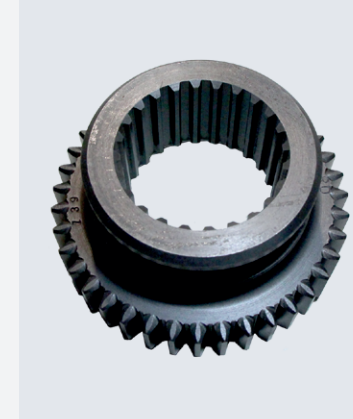
ENGRANAJE TOMA DIRECTA Z=42
